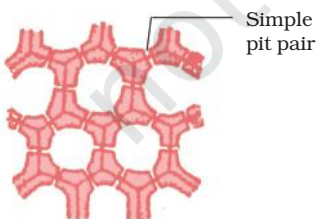
T.S. Sclerenchyma
